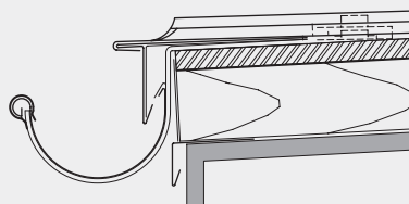
Свес кровли – неправильное исполнение узла
