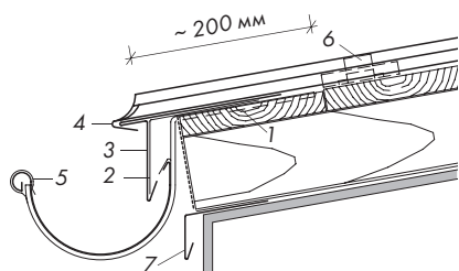
Свес кровли на деревянной обрешетке без ОДМ
