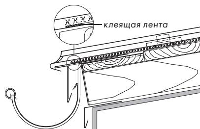
Окончание свеса кровли с ОДМ
