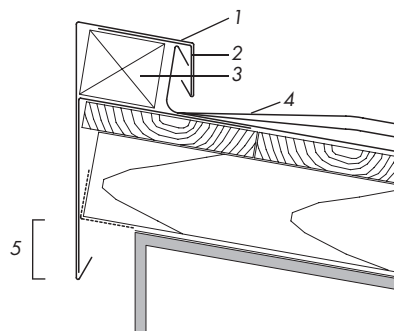
Конек односкатной кровли с брусом кровли
